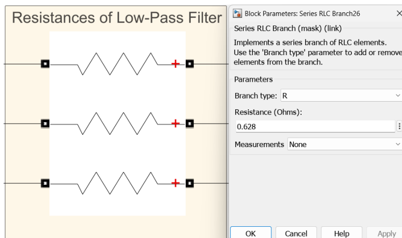
شكل 18: إدخال قيم المقاومات الخاصة بفرع الترشيح
