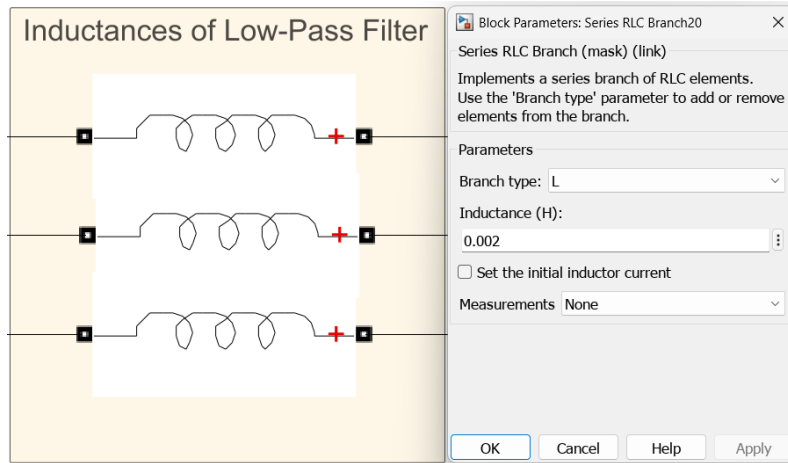
شكل 17: نافذة بارامترات ملفات الخنق في النموذج المطور
