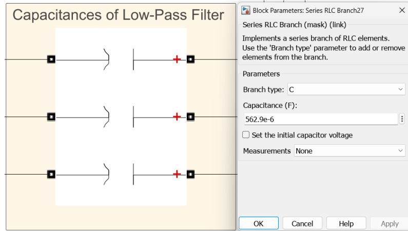
شكل 19: ضبط قيم السعات لمرشح التمرير المنخفض
